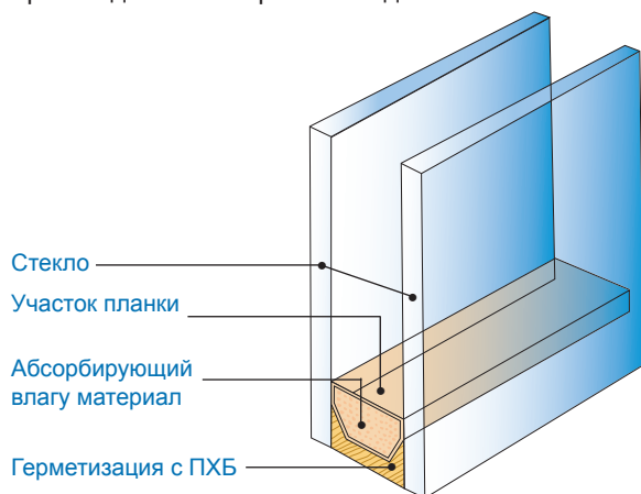
Разрез изолированного оконного стекла
