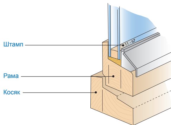
Разрез изолированного оконного стекла со штампом
